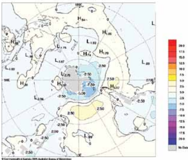
Fig. 8 Summer 2008-09 MSLP anomaly (hPa).
